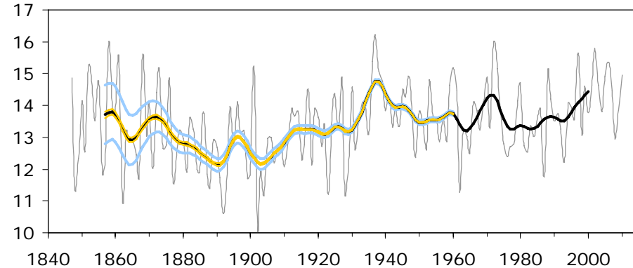
KESÄ 1911-2010: + 0.7 °C
