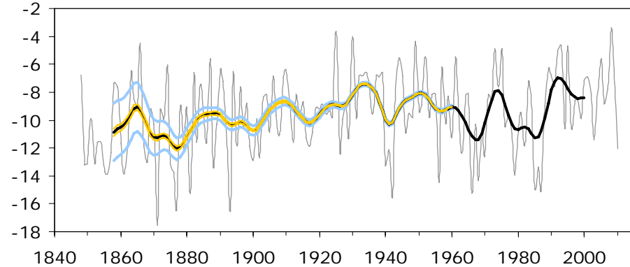
TALVI 1911-2010: + 0.7 °C
