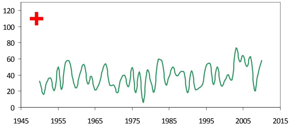
koko Suomi 1950-2010
