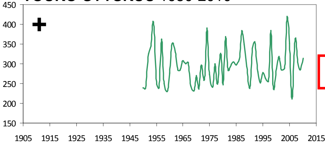
TOUKO-SYYSKUU 1950-2010
