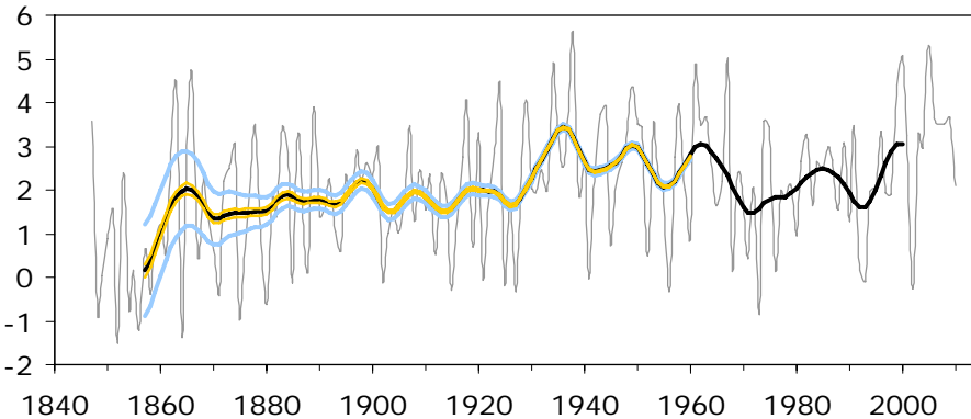
SYKSY 1911-2010: + 0.6 °C
