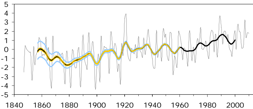
KEVÄT 1911-2010: + 1.7 °C
