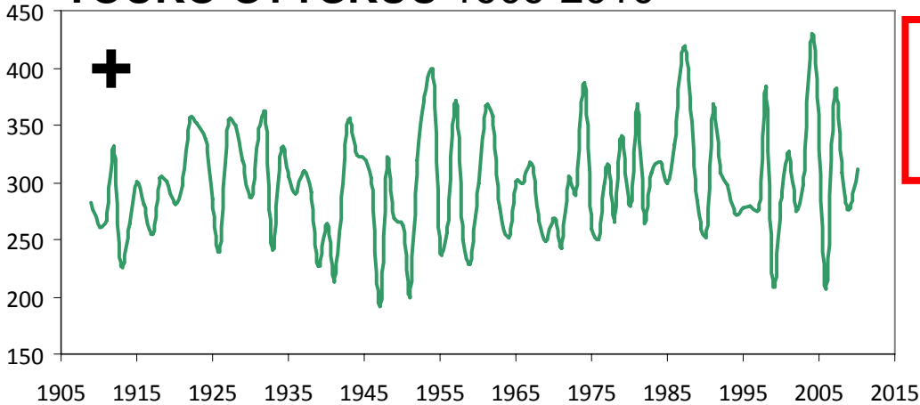
TOUKO-SYYSKUU 1909-2010
